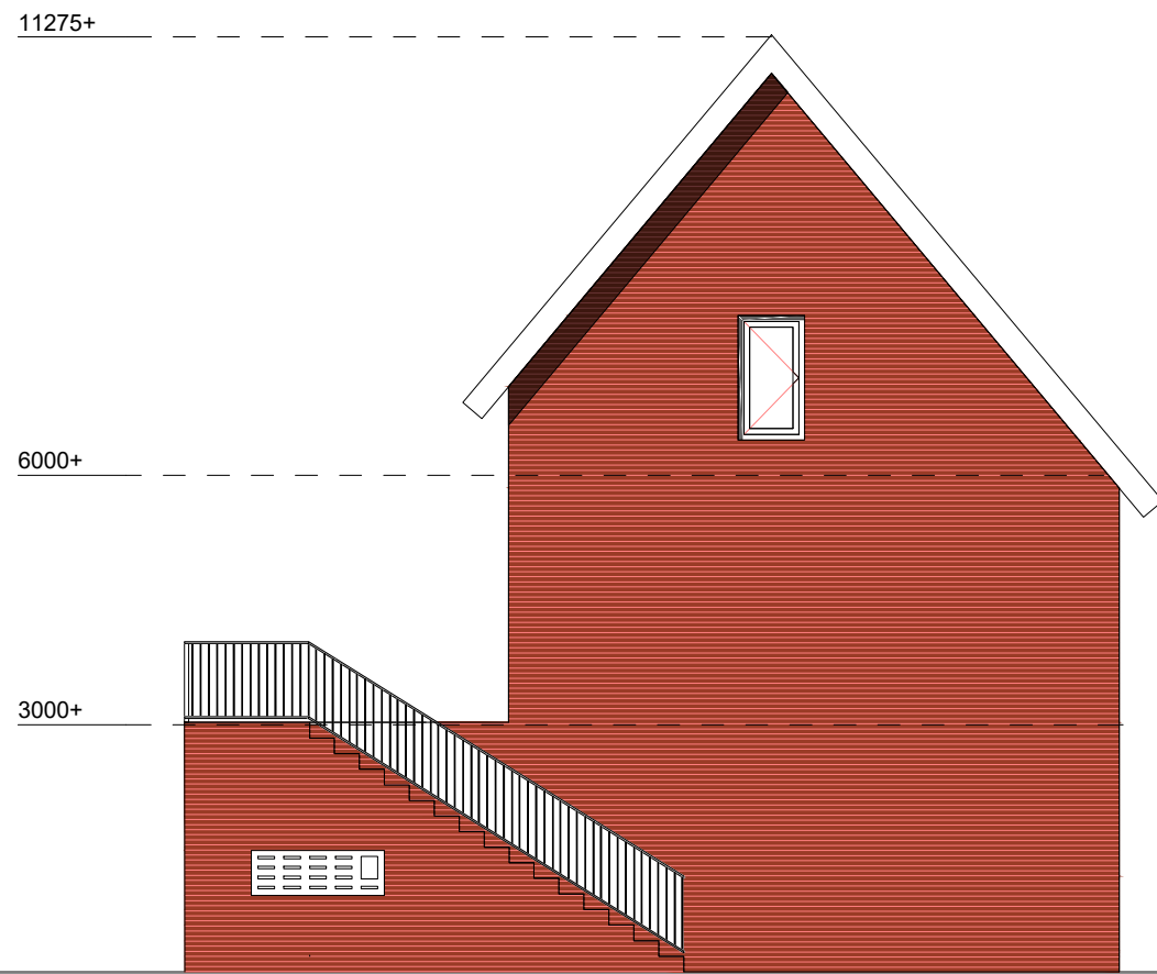
linkergevel
