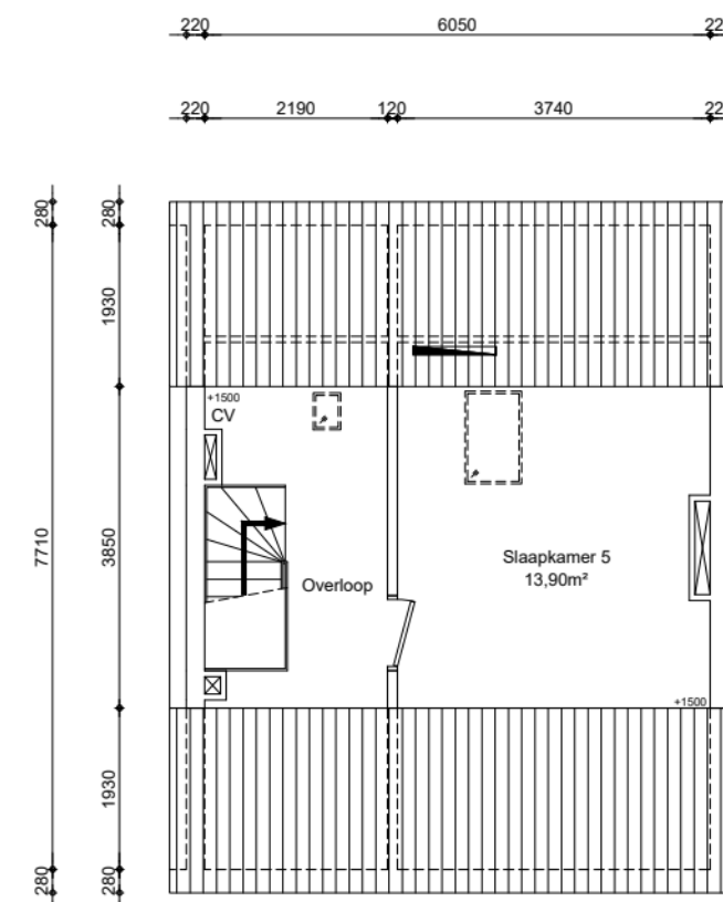
2e verdieping GO wonen 23,29m²
