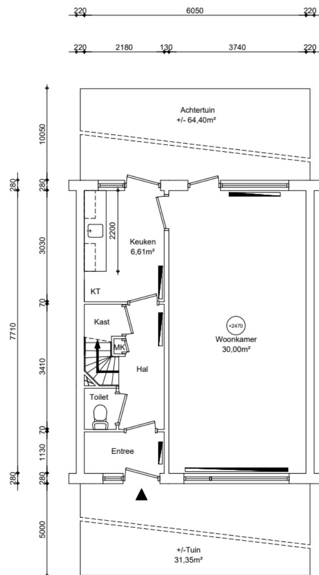
Begane grond GO wonen 46,65m²
