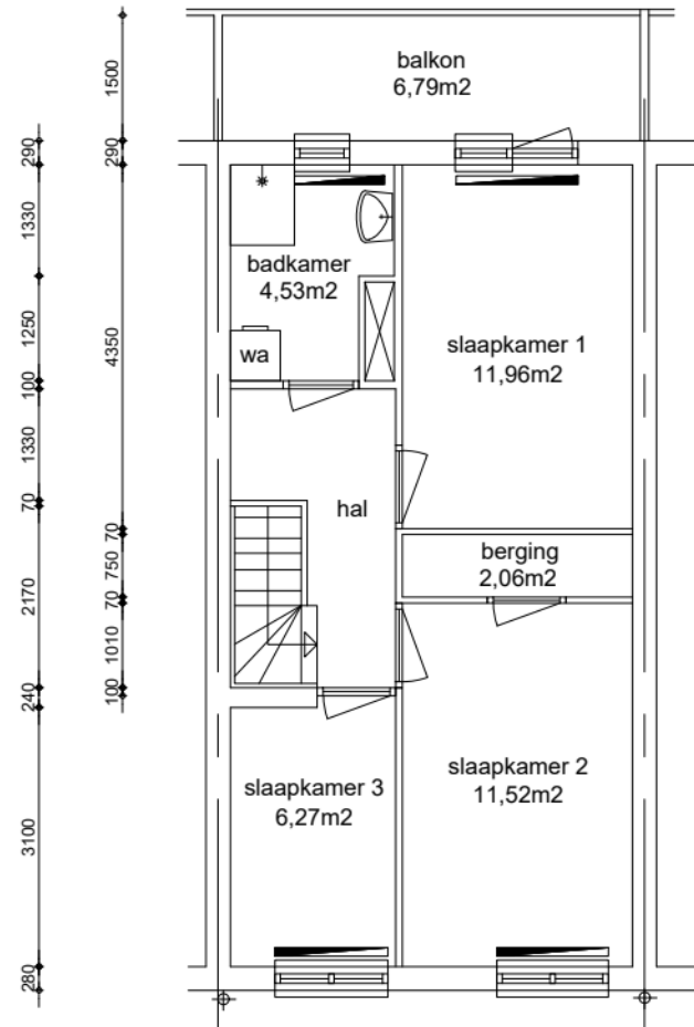
Appartement GO wonen 45,43m²
