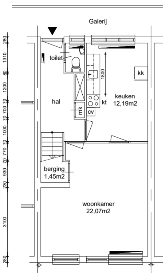
Appartement GO wonen 45,12m²
