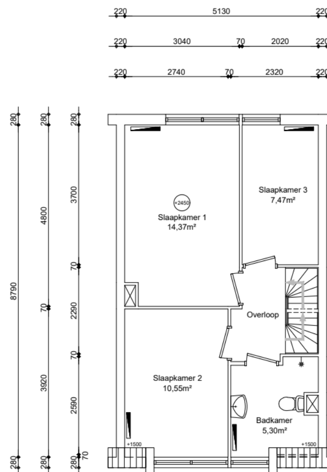
1e verdieping GO wonen 44,57m²
