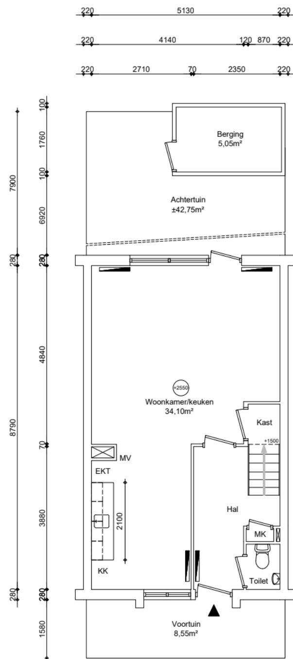
Begane grond GO wonen 45,09m²
