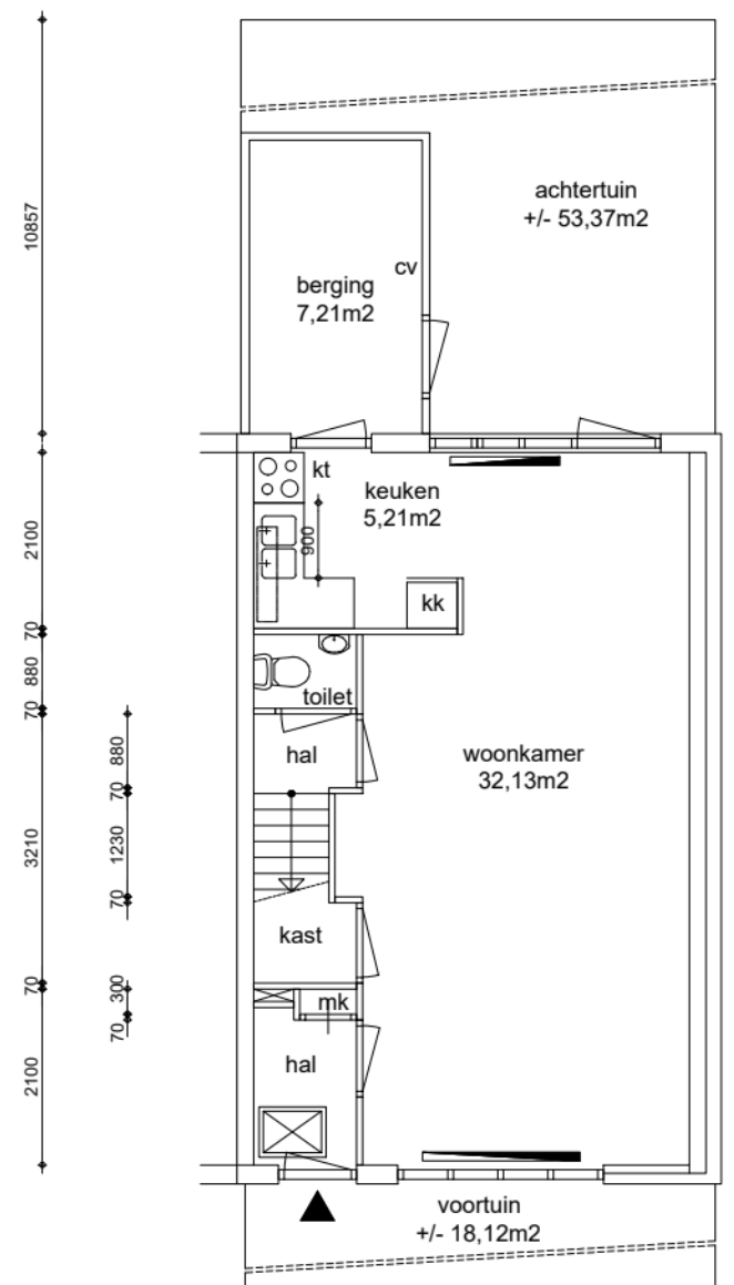
Begane grond GO wonen 51,41m 2
