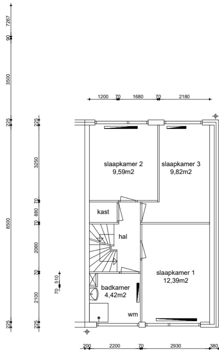
1e verdieping GO wonen 44,20m 2
