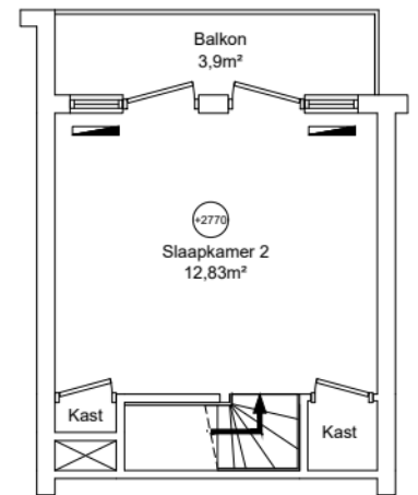
1e verdieping GO wonen 16,41m 2
