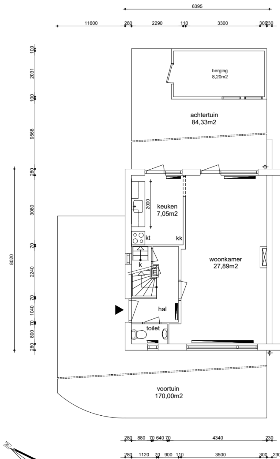
Begane grond GO wonen 44,76m²
