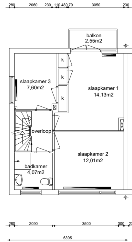
1e verdieping GO wonen 44,64m²
