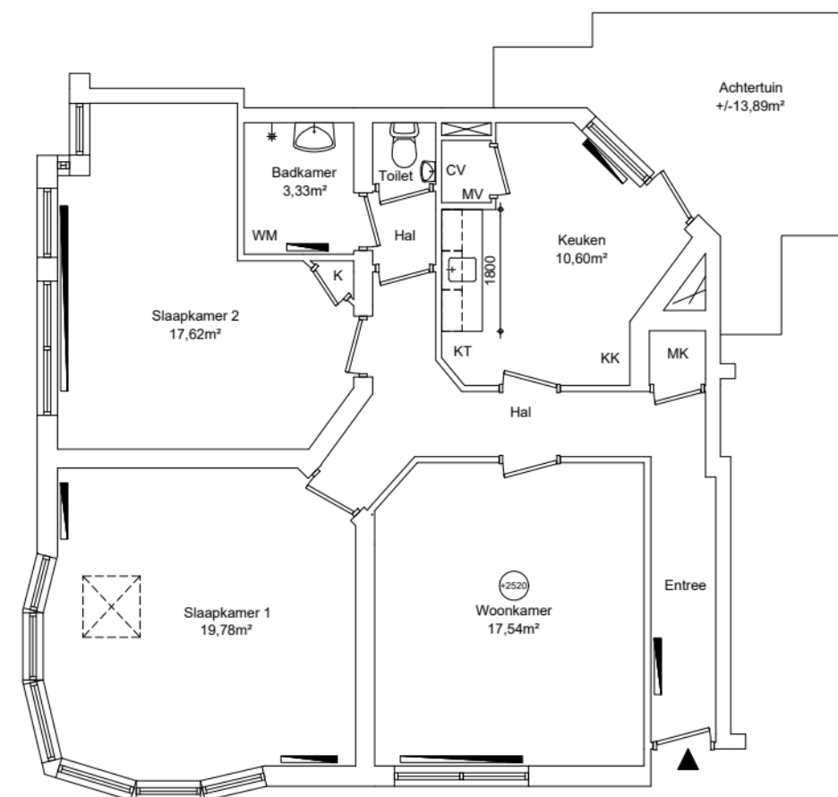
Begane grond GO wonen 85,41m²
