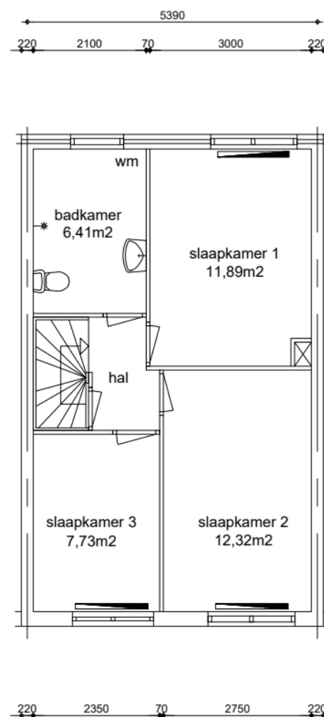
1e verdieping GO wonen 44,36m 2
