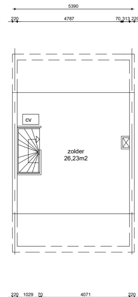
2e verdieping GO wonen 0,00m 2
