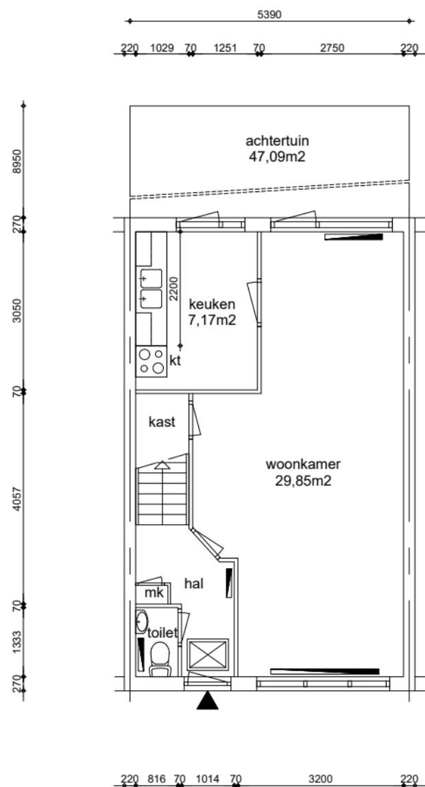
Begane grond GO wonen 44,36m 2
