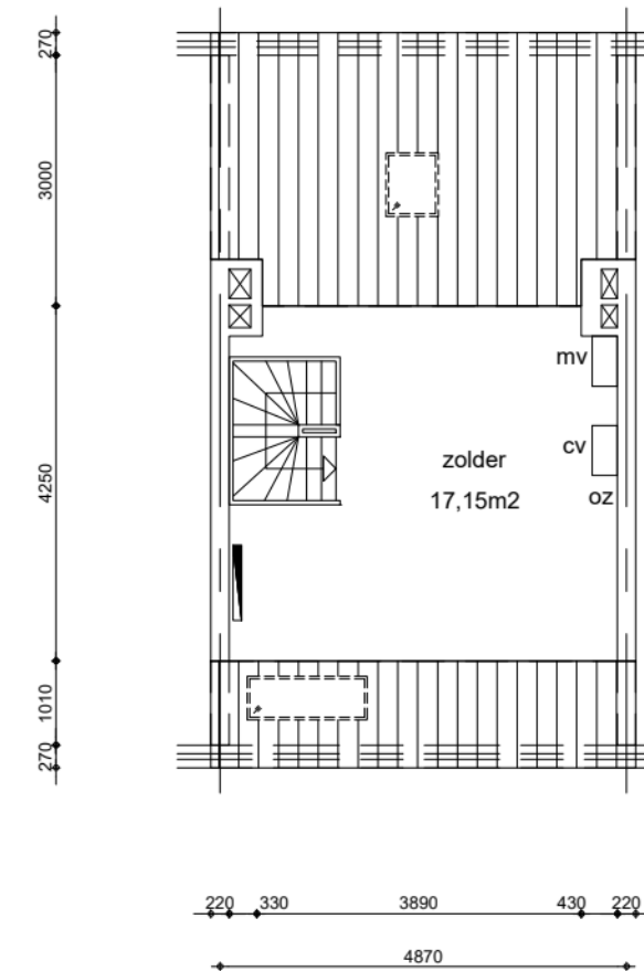
2e verdieping GO wonen 19,76m 2
