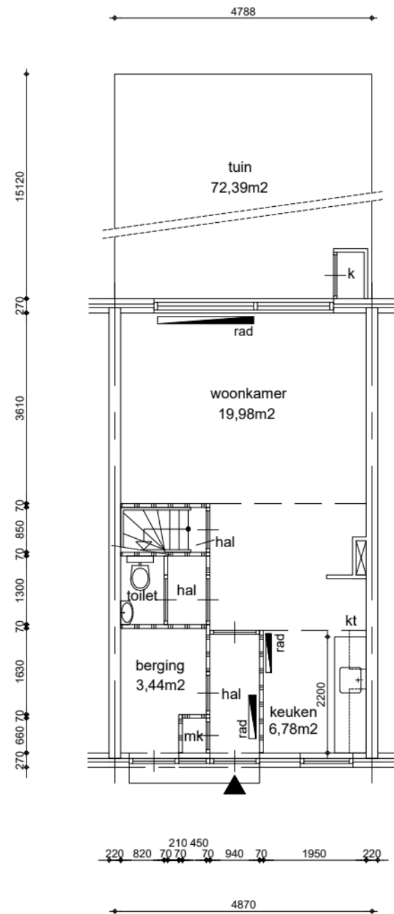
Begane grond GO wonen 38,73m 2
