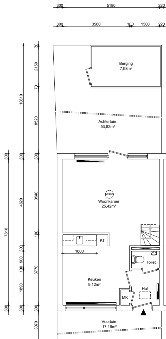
Begane grond GO wonen 40,46m²
