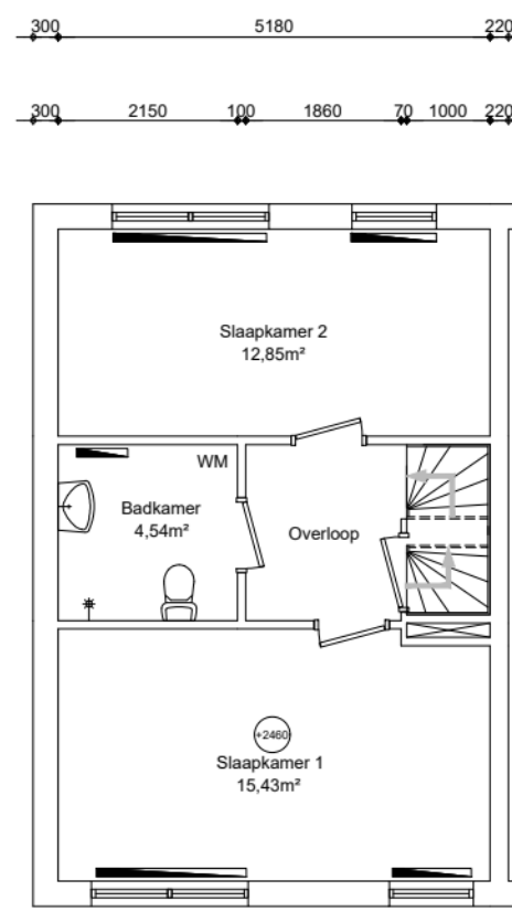
1e verdieping GO wonen 40,46m²
