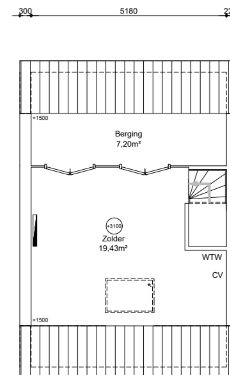
2e verdieping GO wonen 29,16m²
